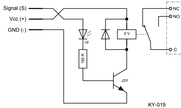
KY-019
